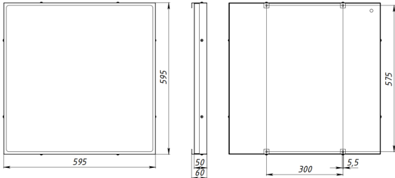
Рисунок 1. Габаритные размеры светильников серии БАЗИС 90Ra IP54.
