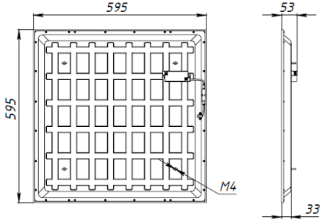
Рисунок 1. Габаритные размеры светильников серии DR9.
