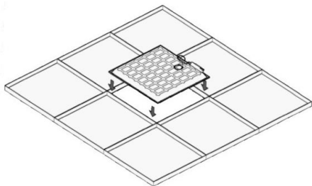
Рисунок 2. Установка в потолок «армстронг».
