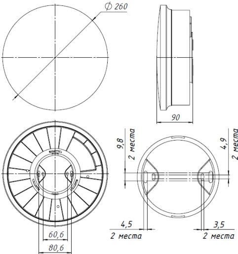
Рисунок 1. Габаритные размеры светильников серии ПОИНТ.
