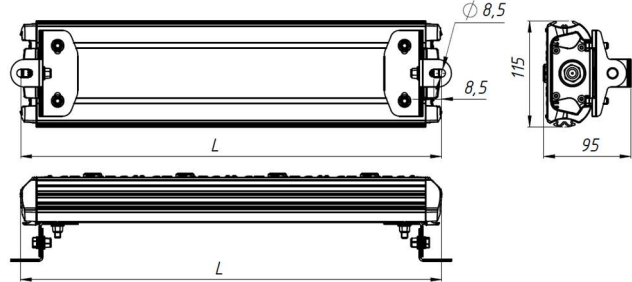
Рисунок 2. Габаритные размеры светильника с креплением.
