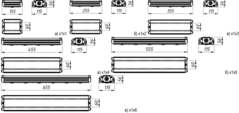
Рисунок 1. Примеры светильников серии ВЕРТО x1.
