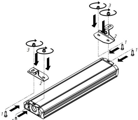
Рисунок 4. Установка крепления на светильник.
