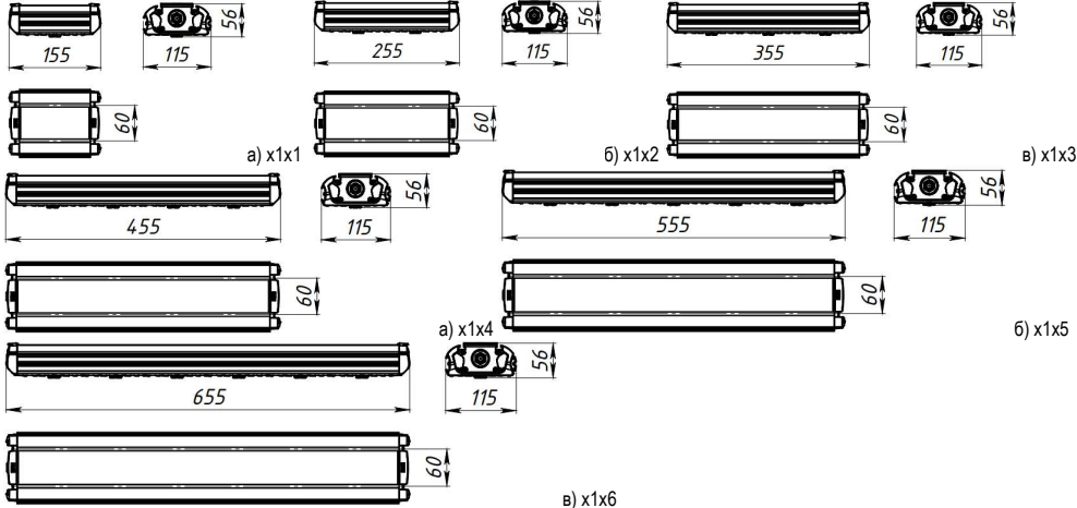
Рисунок 1. Примеры светильников серии ВЕРТО x2.
