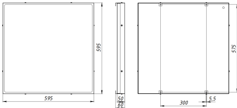
Рисунок 1. Габаритные размеры светильников серии БАЗИС.
